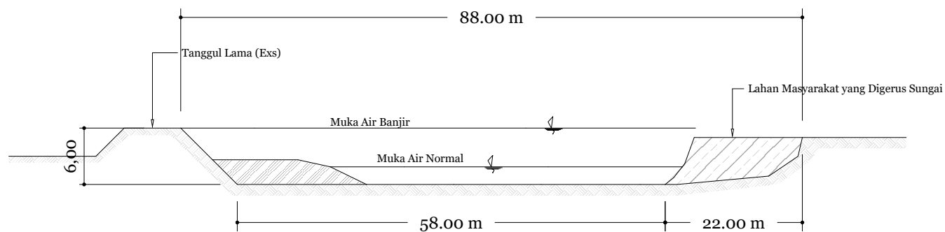
POTONGAN C-C Skala 1:750
