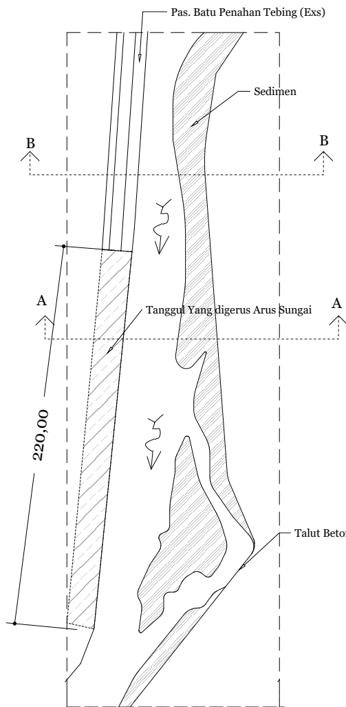
TAMPAK ATAS Skala 1:3000
