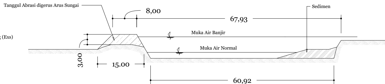
POTONGAN A-A Skala 1:750
