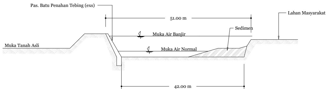
POTONGAN B-B Skala 1:750
