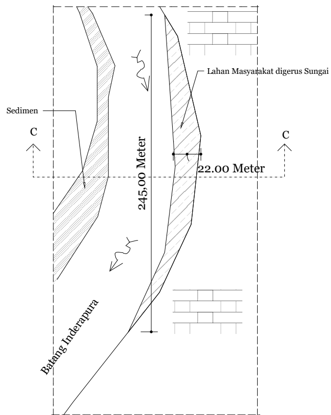
TAMPAK ATAS Skala 1:3000
