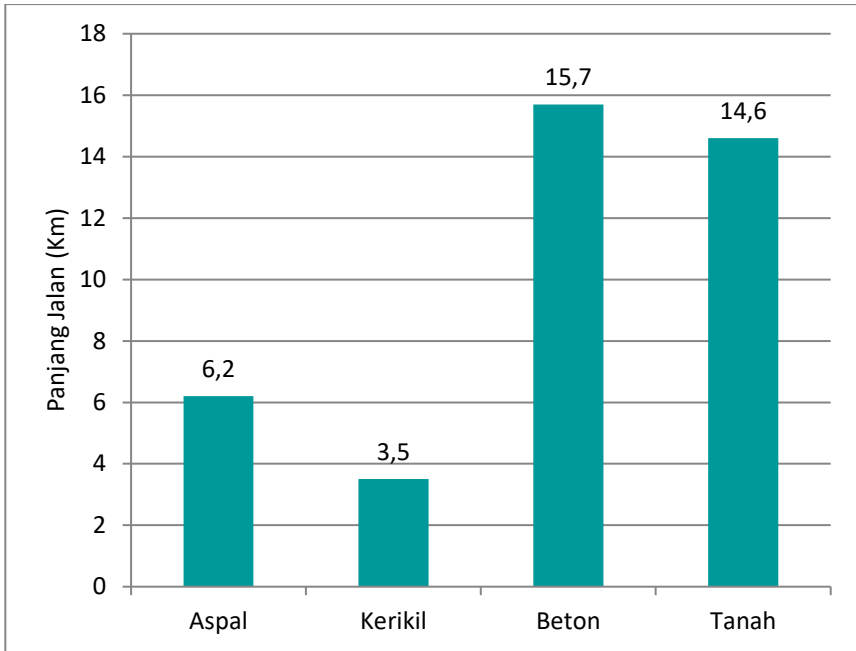
Gambar 6 Panjang Jalan Kabupaten di Kecamatan IV Nagari Bayang Utara Menurut Jenis Permukaan Jalan (Km), 2018
